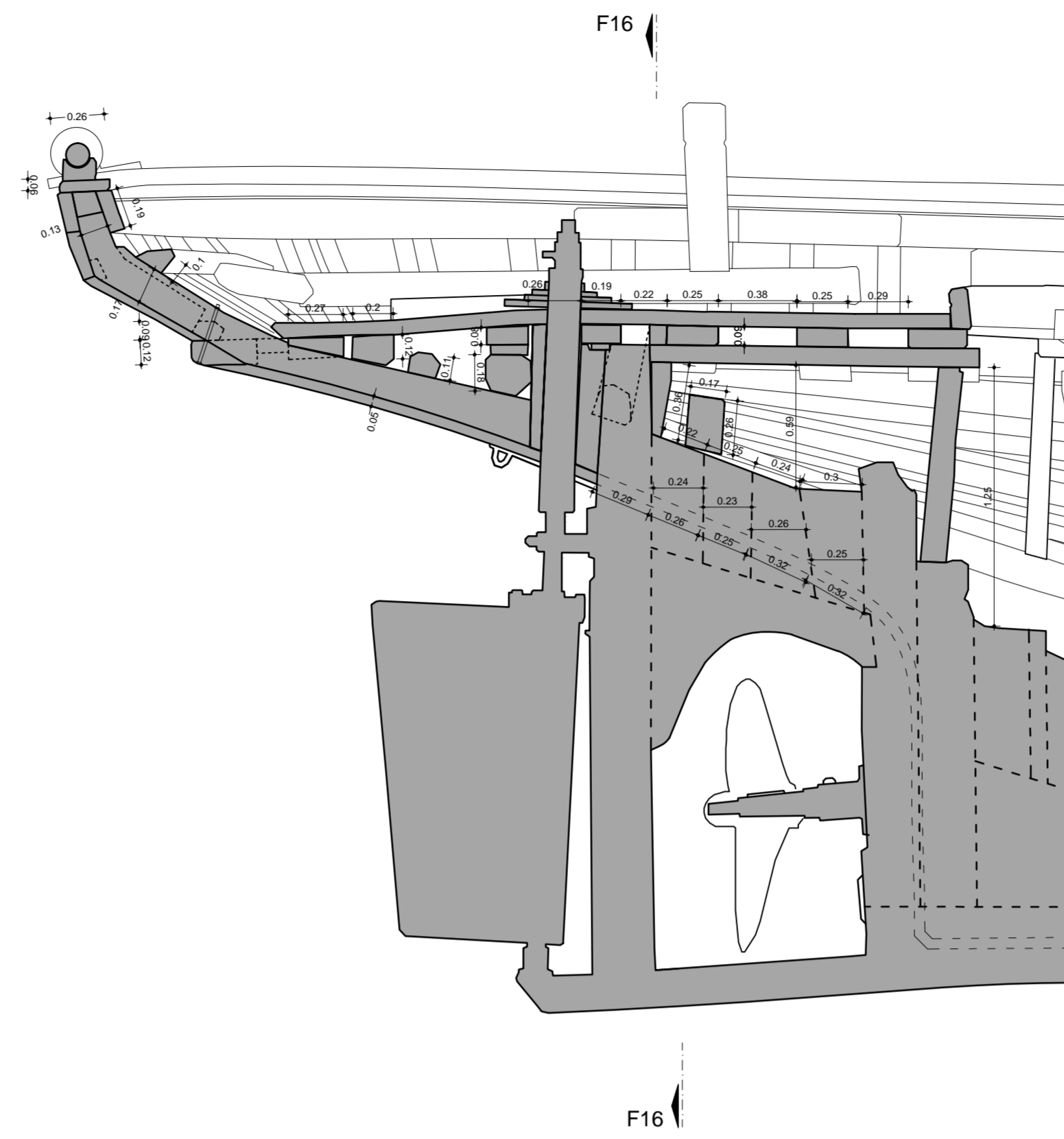
LONGITUDINAL SECTION
